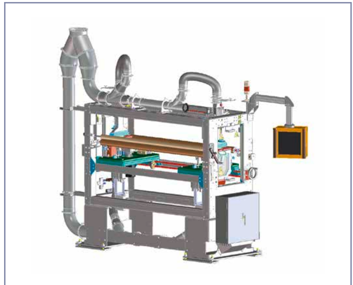
Längstrennsäge mit 2 Aggregaten für Randbeschnitt
